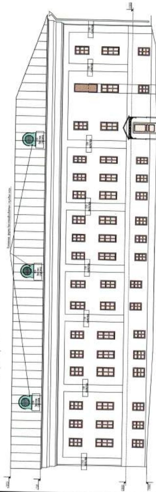
Северный фасад
